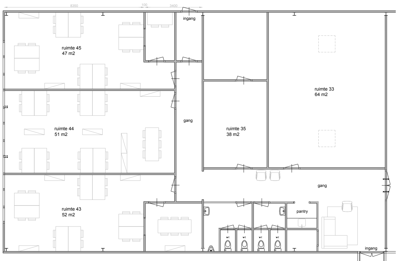
plattegrond eerste verdieping
